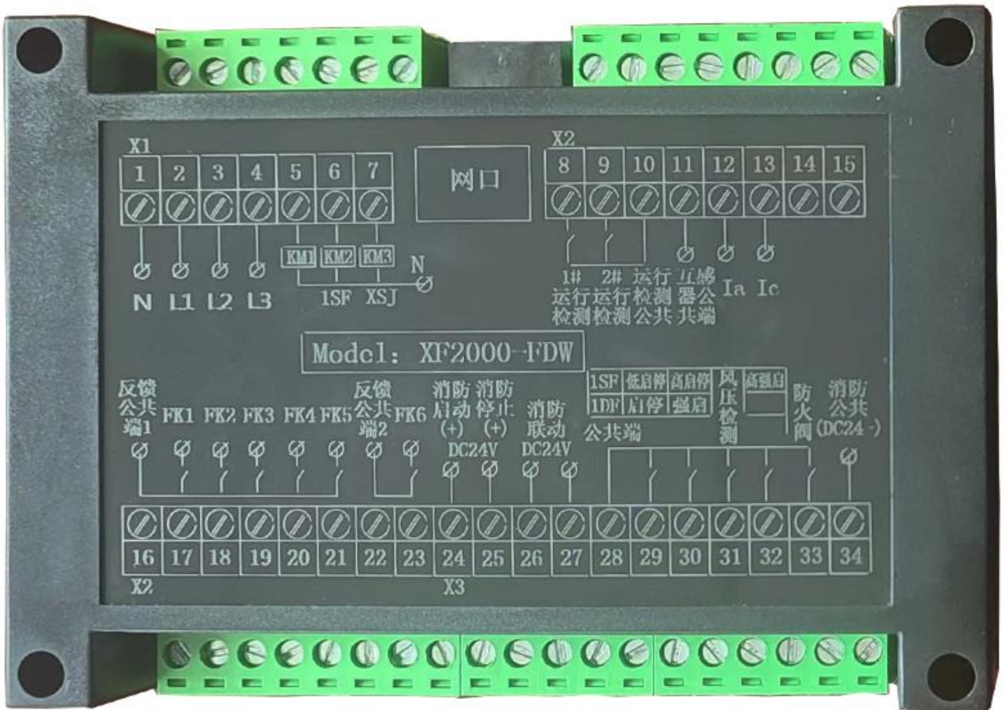
控制器底壳尺寸 145*90*40mm
